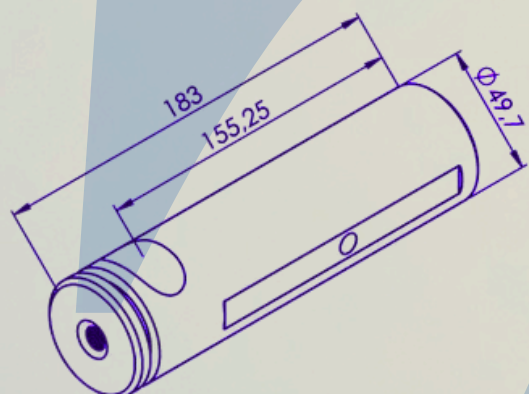
MSU1128 PERNO DE BALANCIN ATEGO Ø50 X 183
