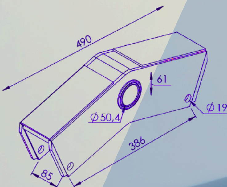
MSU1007/60 BALANCIN MB PARA PERNO Ø60 SUSPENSYS
